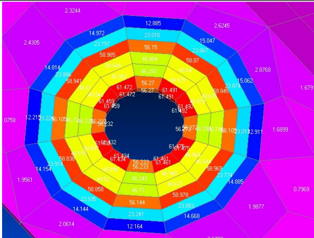
Slika 39. Model 4- Smična naprezanja u donjem laminatu (LC), \sigma_{\max}=70.845 \text{ N/mm}^2
