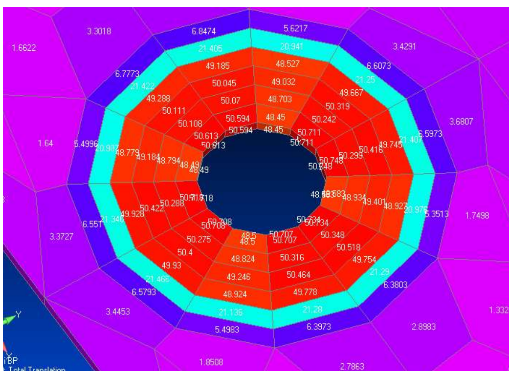
Slika 34. Model 3- Smična naprezanja u gornjem laminatu (LC), \sigma_{\max}=50.708 \text{ N/mm}^2
