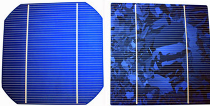
Slika 18. Monokristalna ćelija lijevo i polikristalna desno
