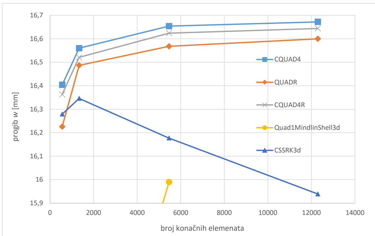
Slika 27 Uvećani detalj zajedničkog prikaza konvergencije rješenja modela dvodna
