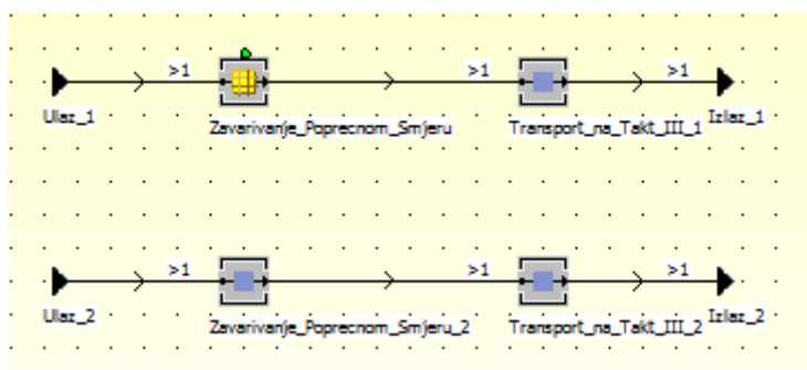
Slika 23. Drugi takt radionice podsklopova
