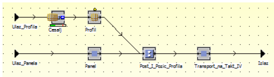
Slika 30. Treći takt radionica ravnih plošnih sekcija
