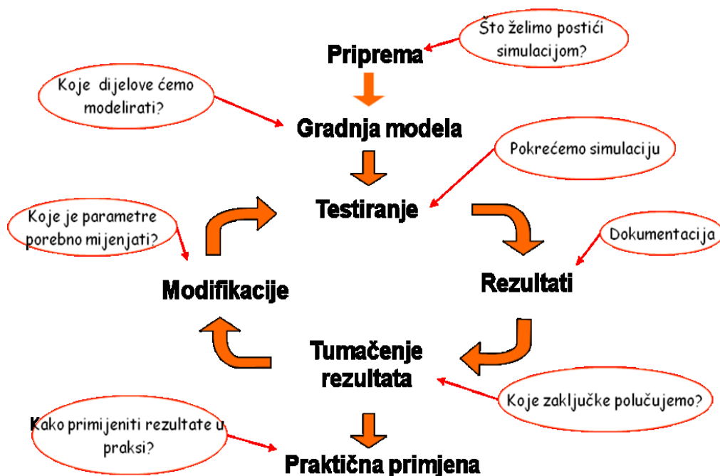
Slika 5. Stvaranje simulacije
