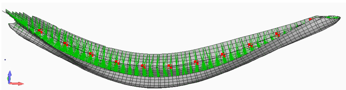
Slika 12. MKE model broda 4 (1. oblik vibriranja)
