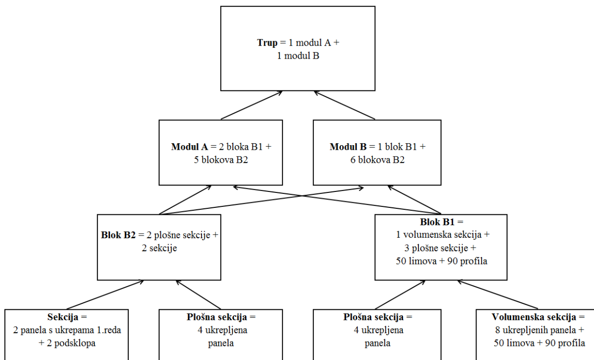
Slika 1. Shema nastanka trupa samopodizne platforme
