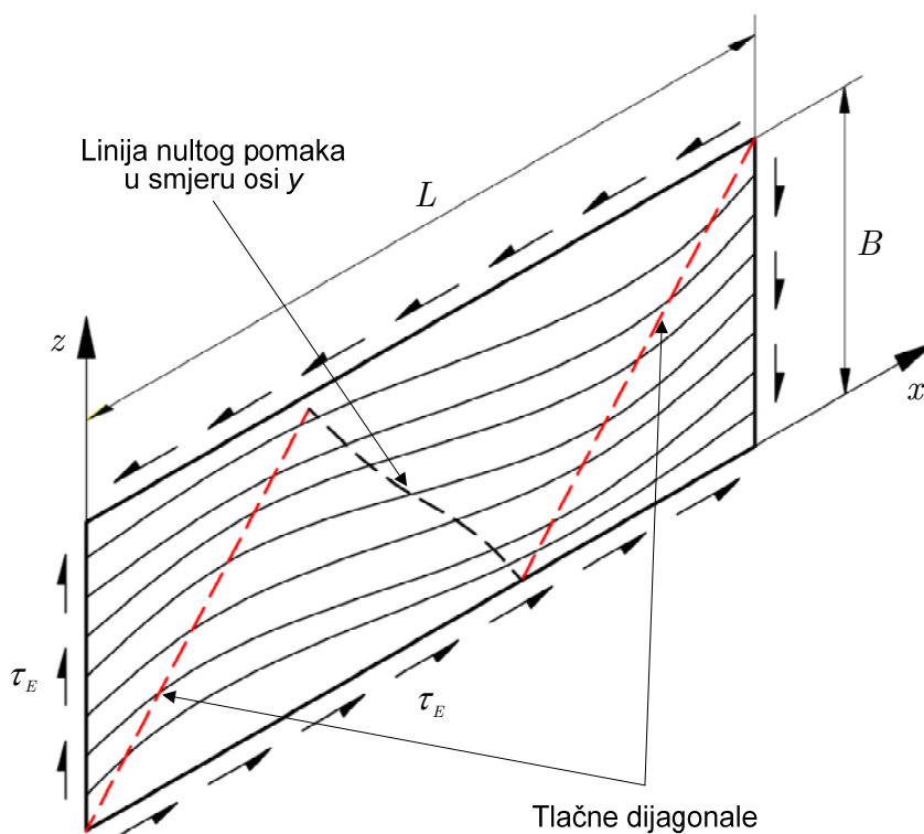
Slika 1. Smično izvijanje zglobno oslonjene ploče.
