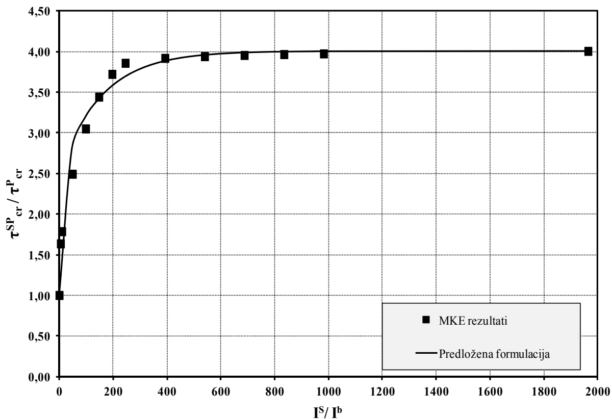
Slika 18. Povećanje kritičnog smičnog napreznja za razmatrani panel AR3-T16-S1L.
