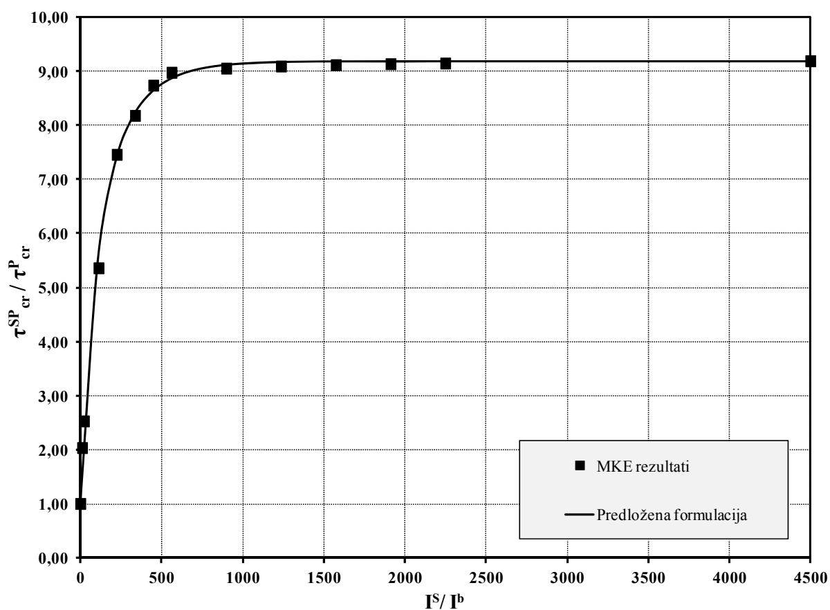
Slika 19. Povećanje kritičnog smičnog napreznja za razmatrani panel AR3-T16-S2L.
