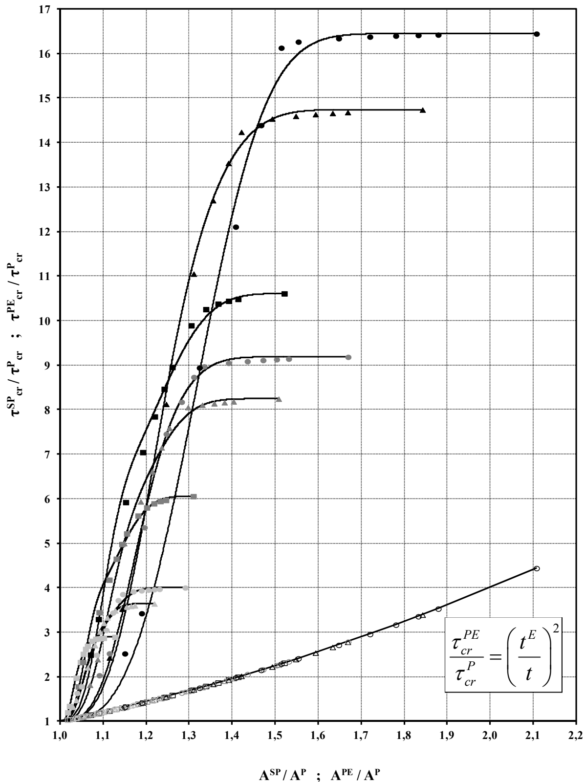
Slika 21. Zbirni dijagram povećanja kritičnog smičnog napreznja svih razmatranih panela u ovisnosti o povećanju površine poprečnog presjeka.
