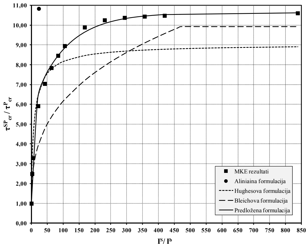
Slika 14. Povećanje kritičnog smičnog napreznja za razmatrani panel AR1-T16-S3L.
