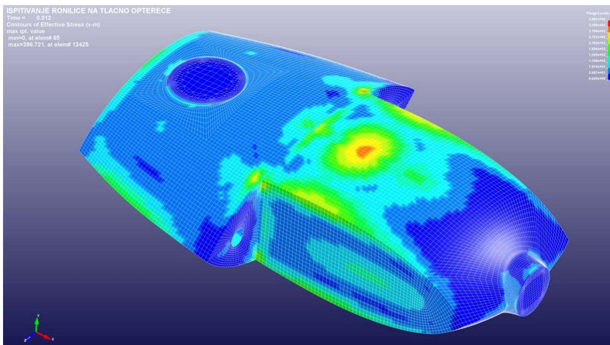
Slika 55 – Polje von Mises naprezanja ronilice za slučaj 2
