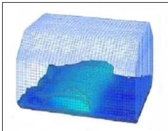
Slika 3.4. CFD simulacija – nisko punjenje [2]
