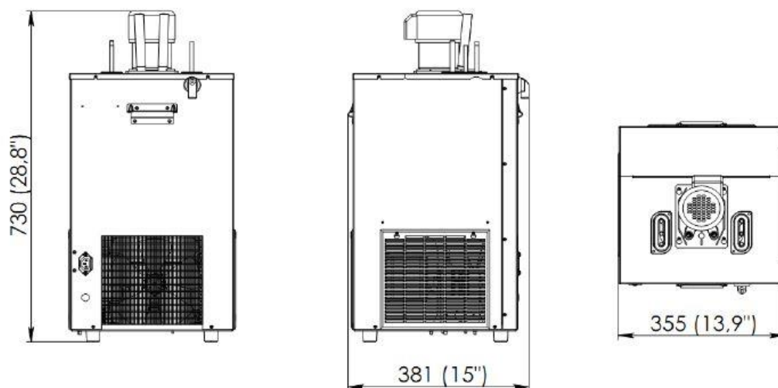
Slika 22. UBC Tayfun-75
