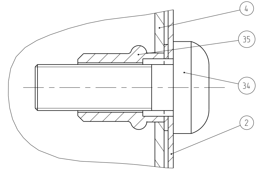
Detalj A M 5:1
