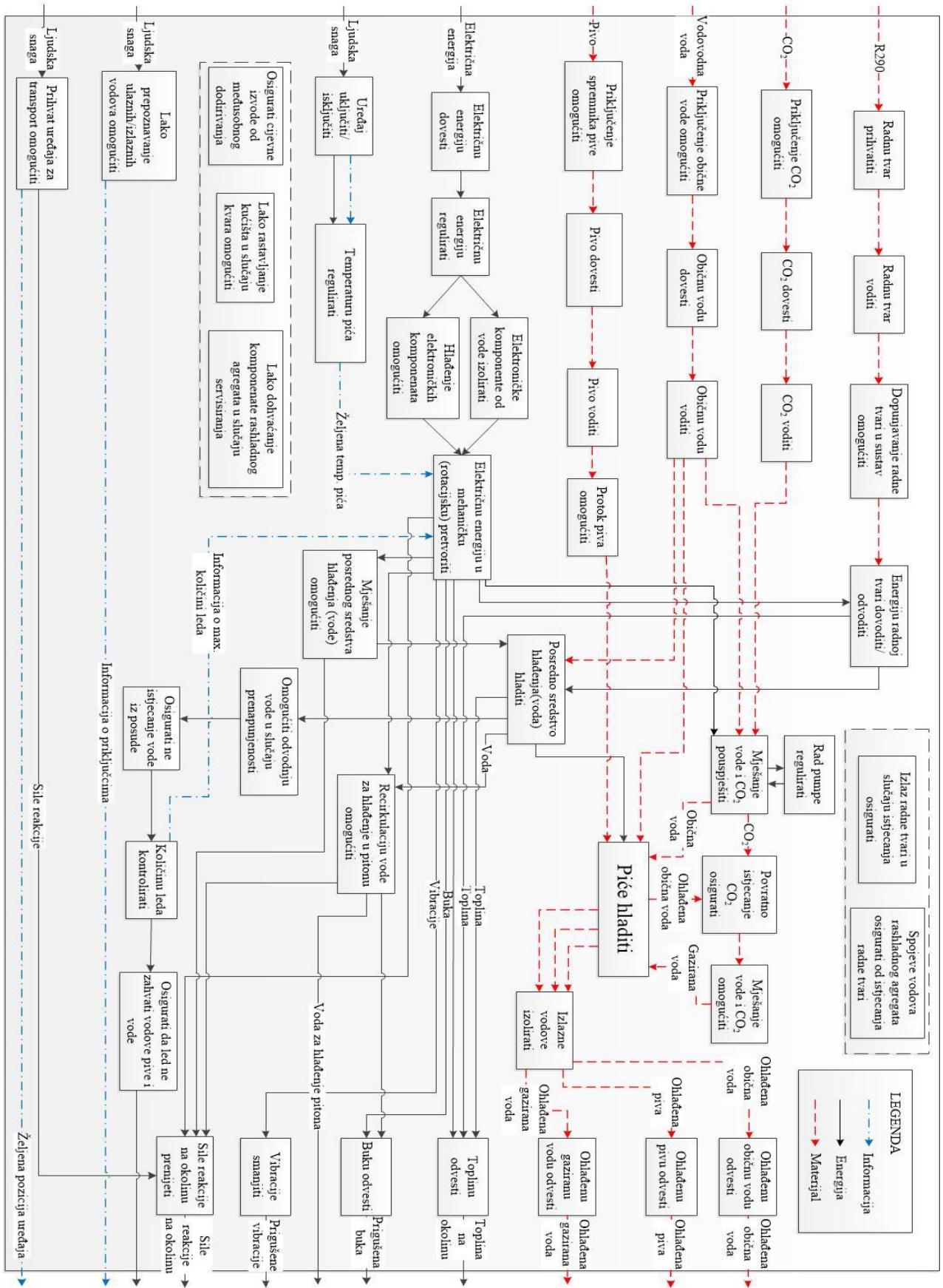
Slika 34. Funkcijska dekompozicija
