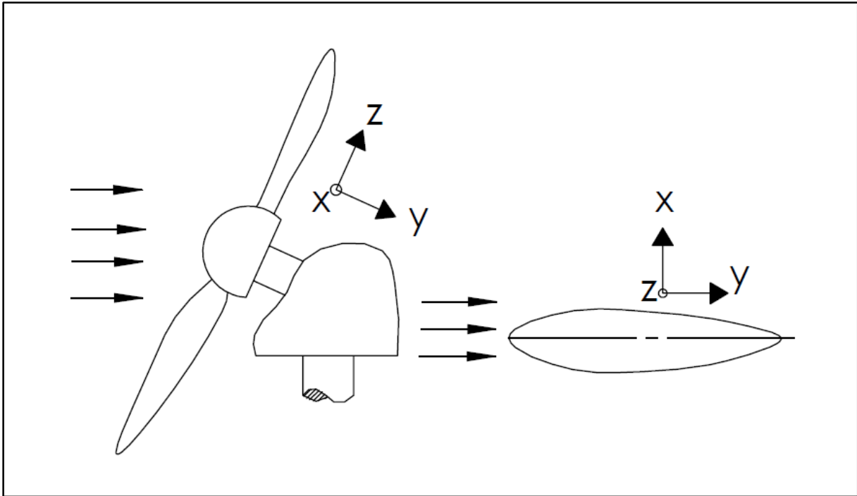
Slika 10. Koordinatni sustavi
