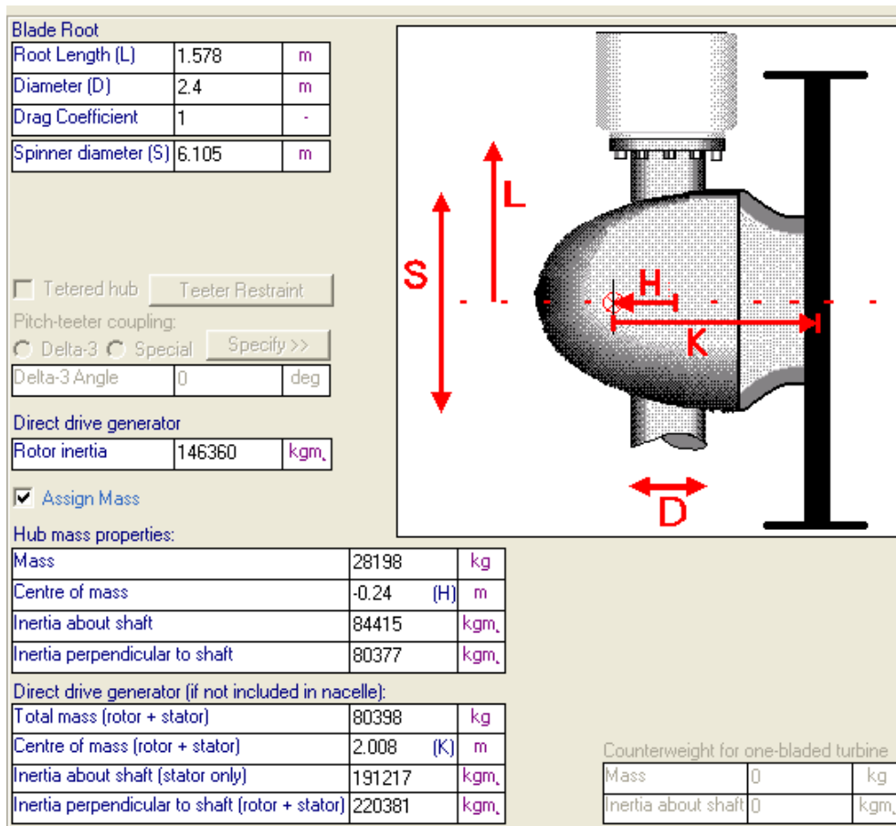
Slika 13. Dimenzije glavčine
