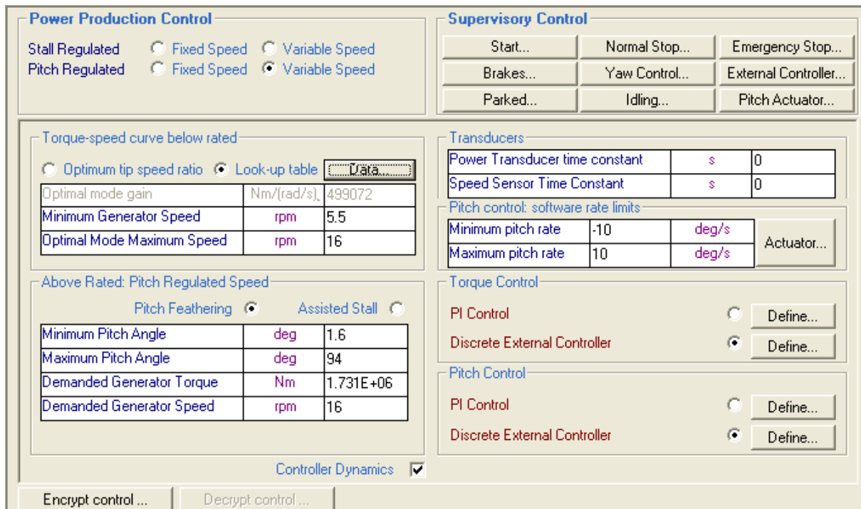
Slika 14. Pitch control
