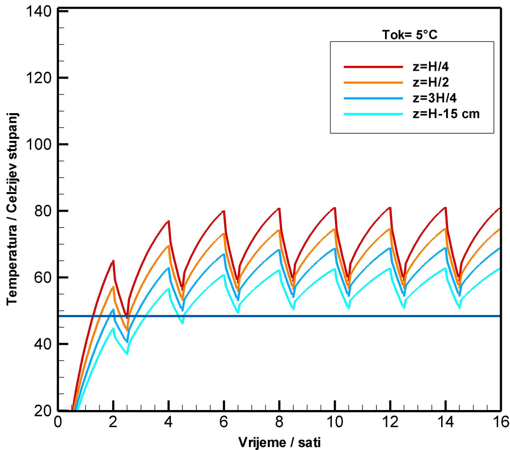
Slika 15. Vremenska promjena temperature unutrašnje površine dimnjaka po njegovoj visini za intermitirajući rad priključnog plinskog trošila ( T_{ok} = 5^{\circ}\text{C} , t_r/t_n = 3 )
