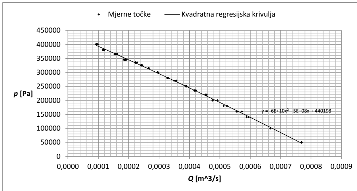
Slika 25. Karakteristika pumpe
