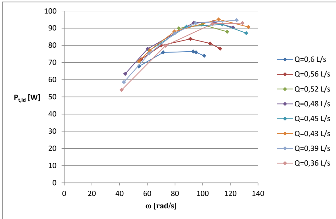
Slika 31. Idealna snaga turbine u ovisnosti o kutnoj brzini
