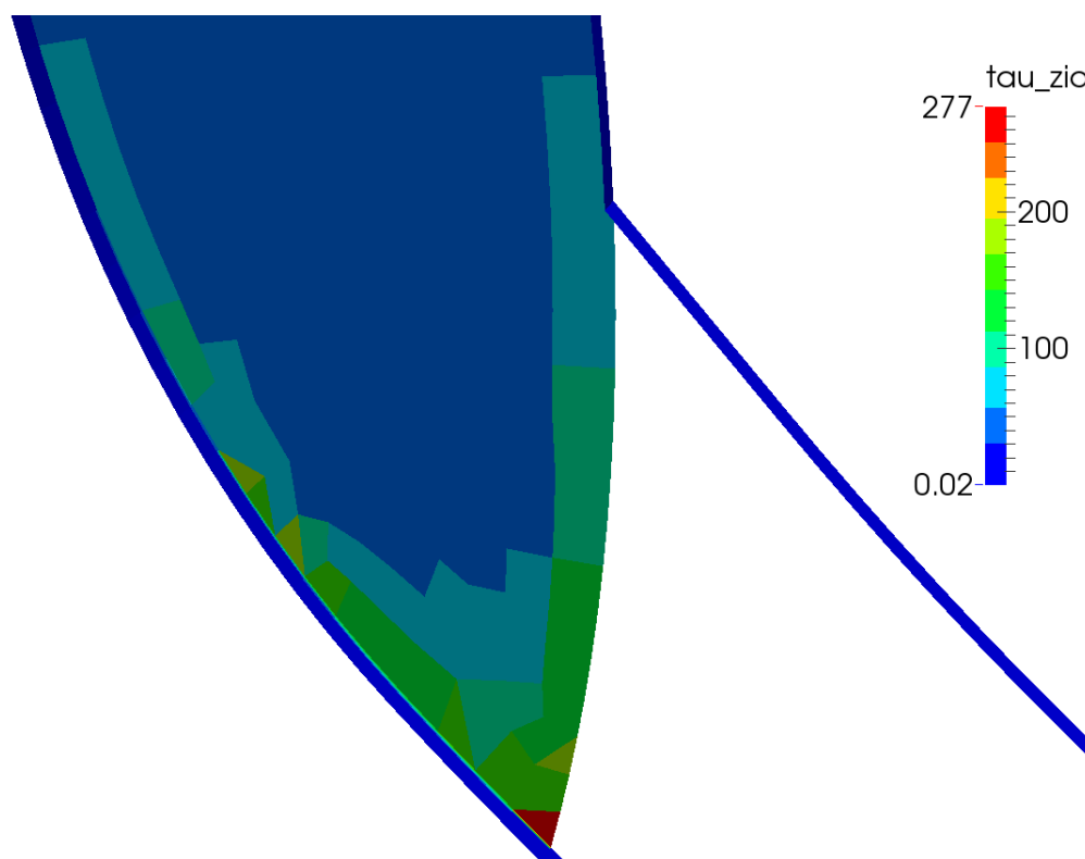
Slika 51. Prikaz polja tangencijalnih naprezanja na detalju spoja ulazne cijevi i diska
