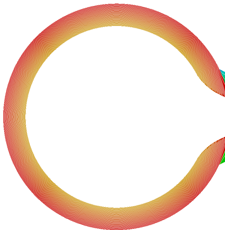
Slika 45. Prikaz strujnica na rotirajućem disku
