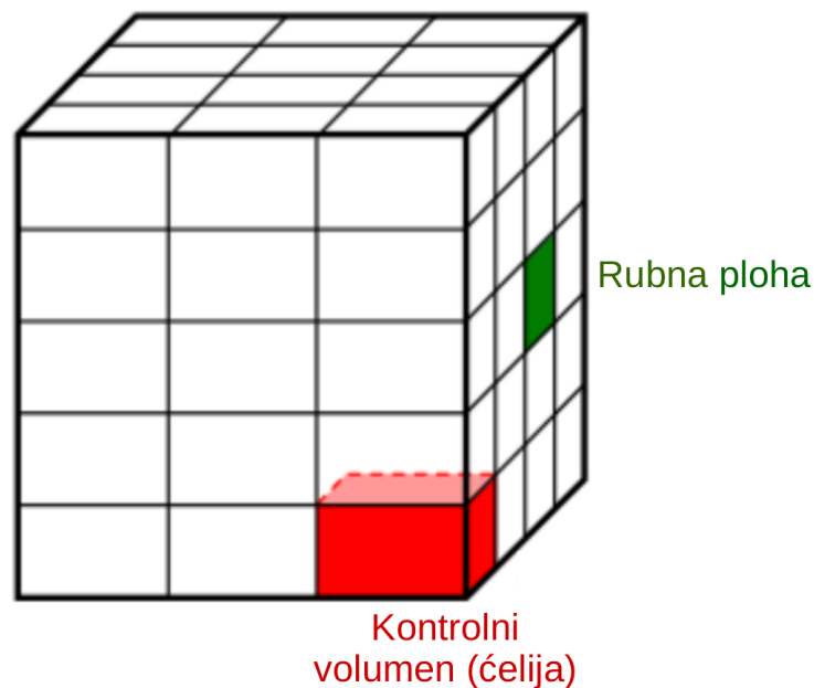
Slika 5. Primjer jednostavne 3D mreže
