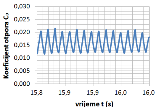
Slika 7.23 C_D pri \alpha=0^\circ (viši red točnosti)
