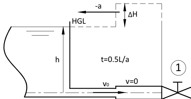
Slika 2. Sustav spremnik-cjevovod u vremenskom trenutku t=0.5L/a
