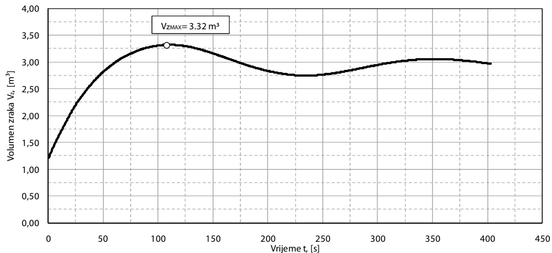
Dijagram 16. Grafički prikaz promjene volumena zraka u tlačnoj posudi
