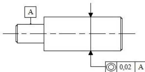
Slika 14. Tolerancija položaja
