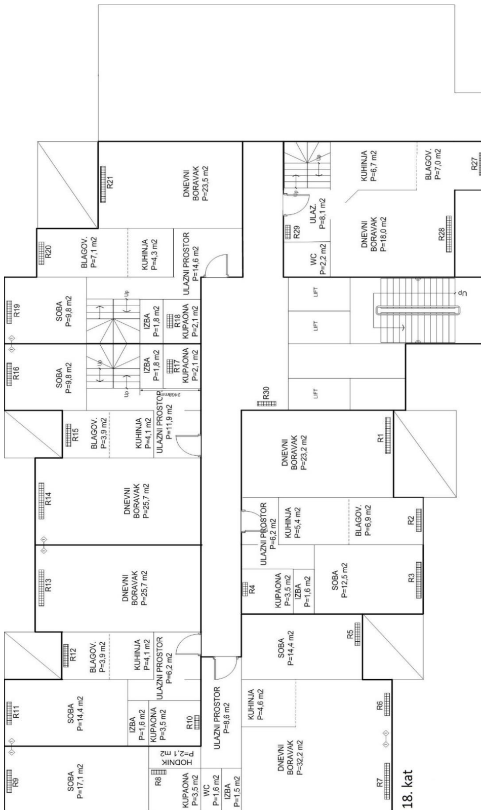
Slika 26 Tlocrt osmog ulaza Mamutica, 18. kat
