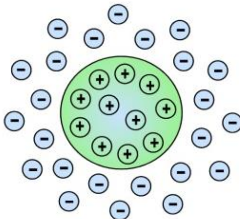
Slika 16. Elektrostatička stabilizacija [25]
