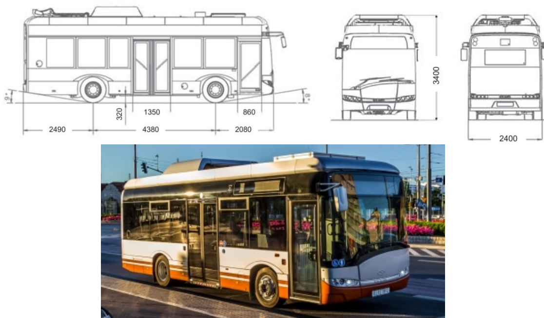
Slika 3.16. Solaris Urbino 8.9 LE [22.]
