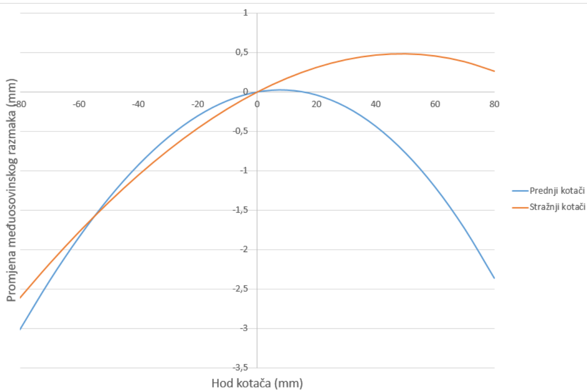
Slika 5.4. Ovisnost međuosovinskog razmaka i hoda kotača
