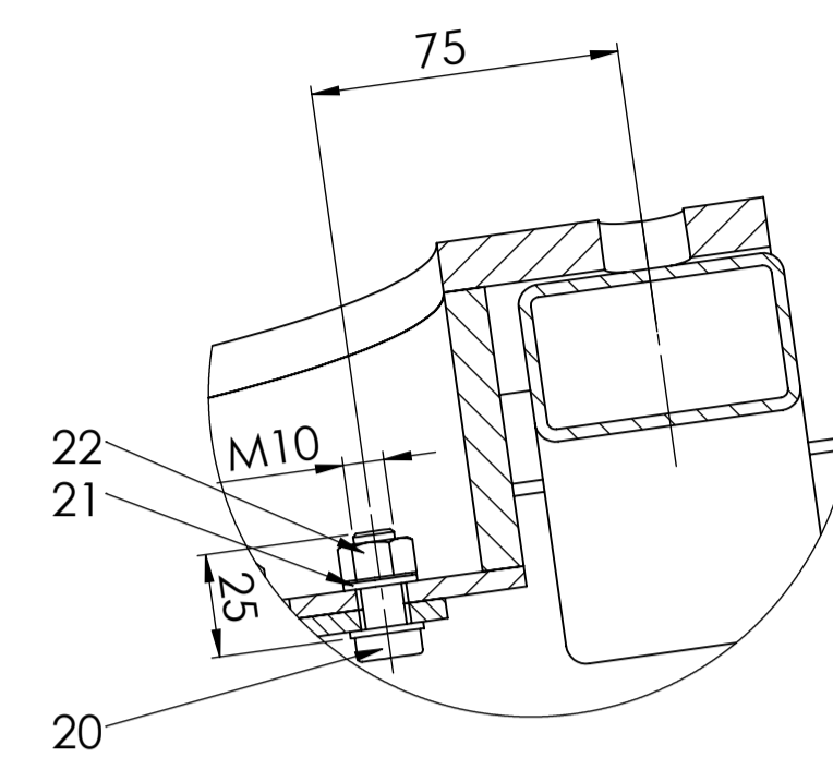
DETALJ J MJERILO 1 : 2
