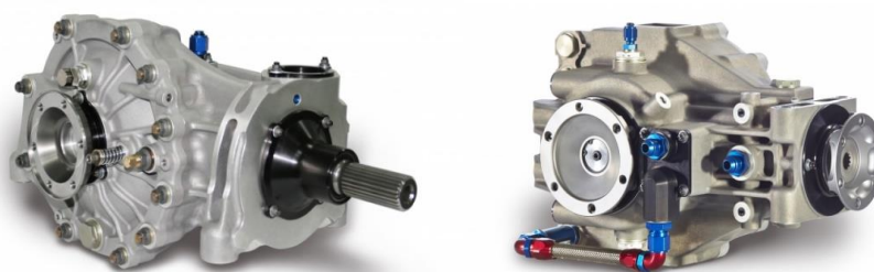
Slika 4.24. X-track diferencijali [43.]
