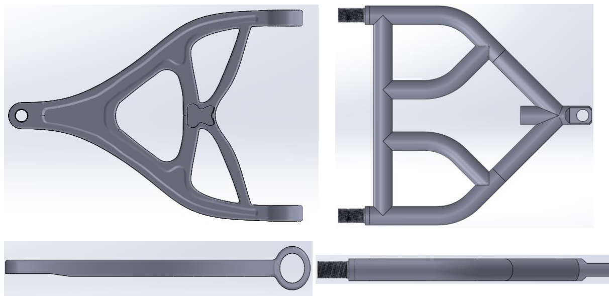
Slika 7.4. Prikaz 3D modela lijevane izvedbe (desno) i zavarene izvedbe s krajcima (desno) donjeg poprečnog ramena
