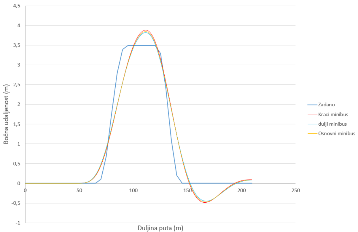
Slika 2.14. Odstupanje vozila različite konfiguracije duljine od zadane putanje kod DLC ispitne procedure
