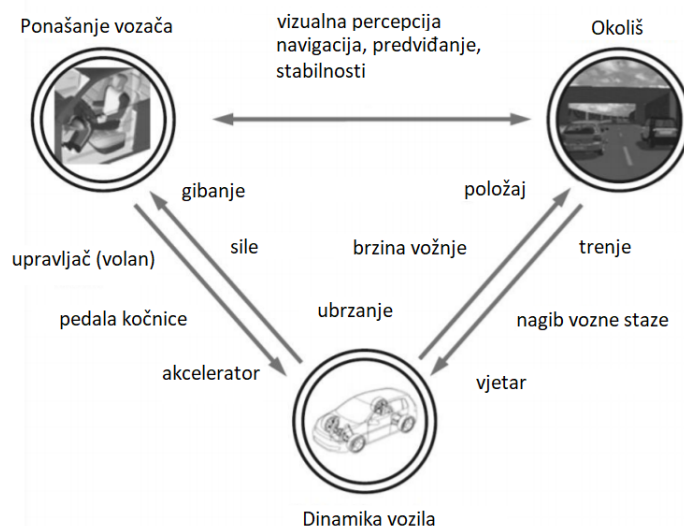
Slika 2.1. Dinamika vozila [6.]
