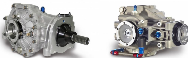
Slika 4.24. X-track diferencijali [43.]
