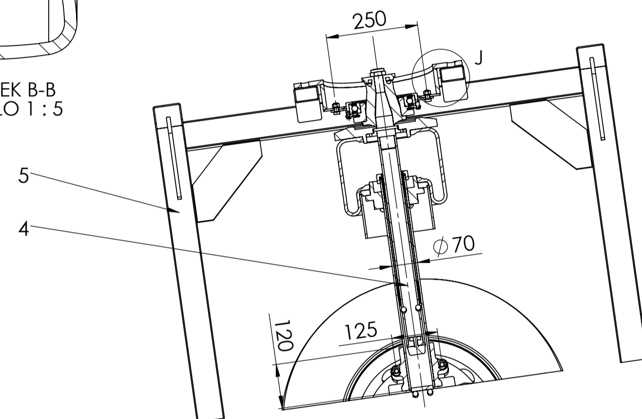
PRESJEK I-I MJERILO 1 : 10
