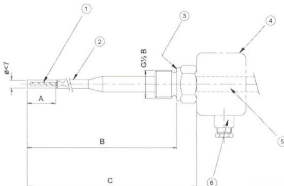
Slika 9. Dimenzije mjerila temperature tipa DL
