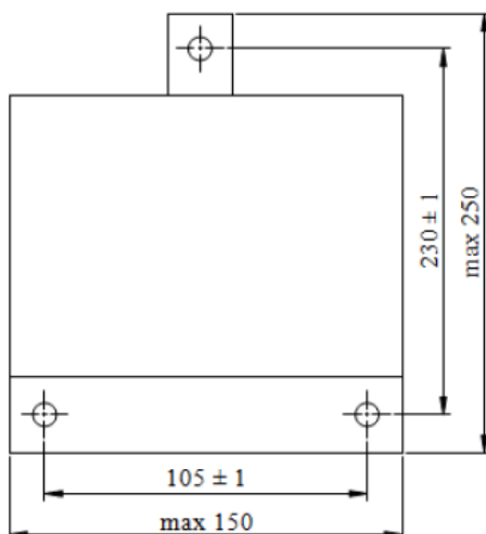
Slika 13. Dimenzije kućišta računске jedinice
