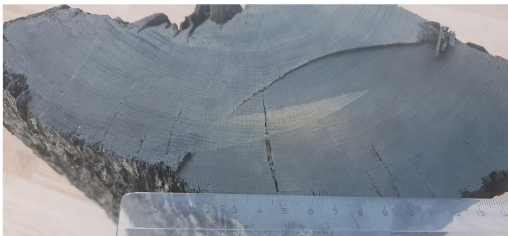
Slika 34. Makrostruktura poprečnog presjeka 1840 godina starog hrasta
