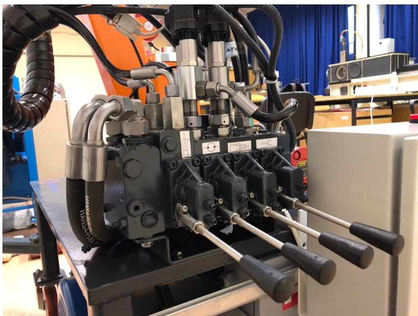
Slika 2. Proporcionalni ventilski blok s označenim segmentima
