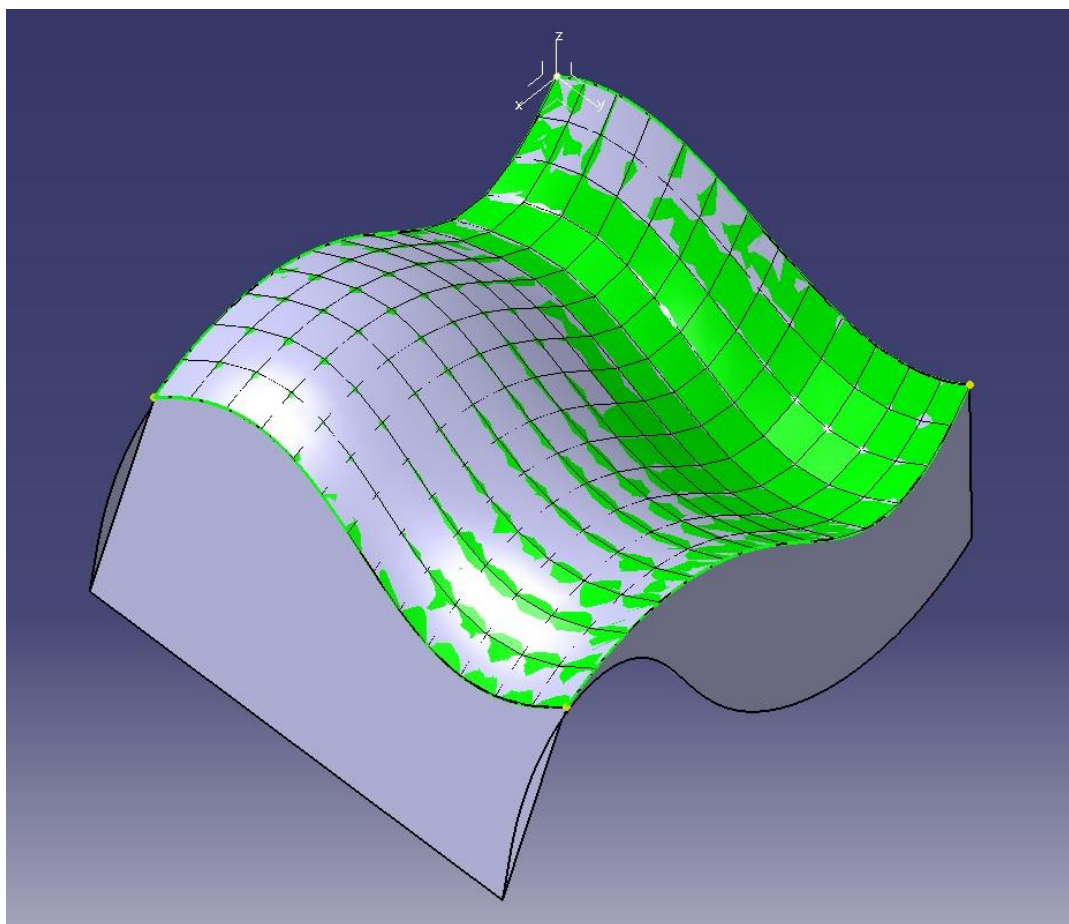
Slika 9. "Mesh-irana" površina
