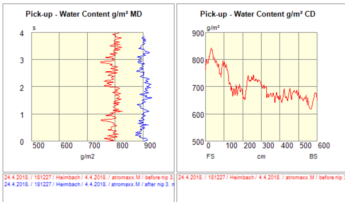
Slika 74. Pick-up ponovljeno, treće mjerenje, MD i CD količina vode
