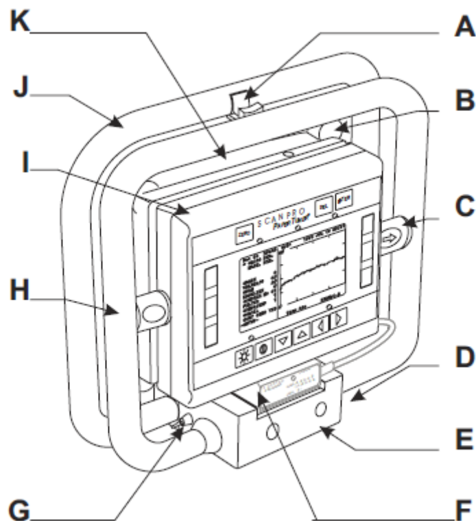
Slika 15. Skica uređaja ScanPro [9]
