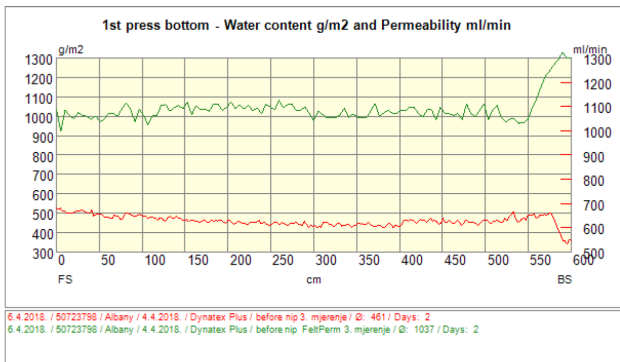
Slika 63. Prvi donji filc, treće mjerenje, CD količina vode i propusnost
