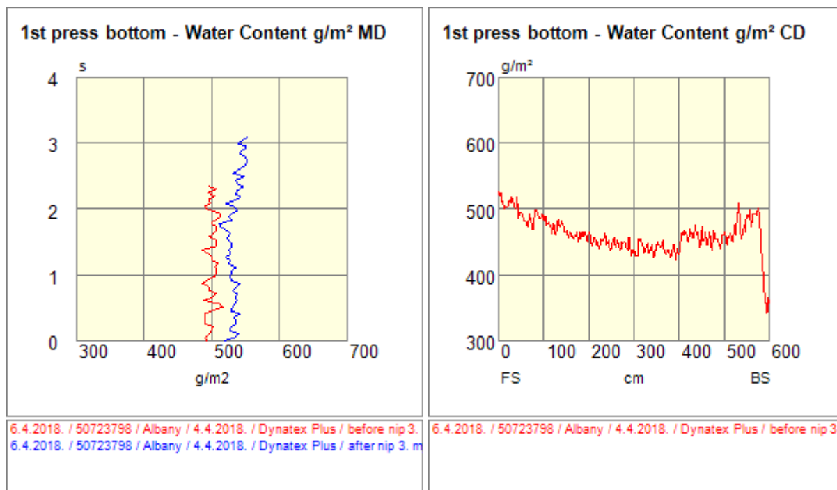
Slika 62. Prvi donji filc, treće mjerenje, MD i CD količina vode
