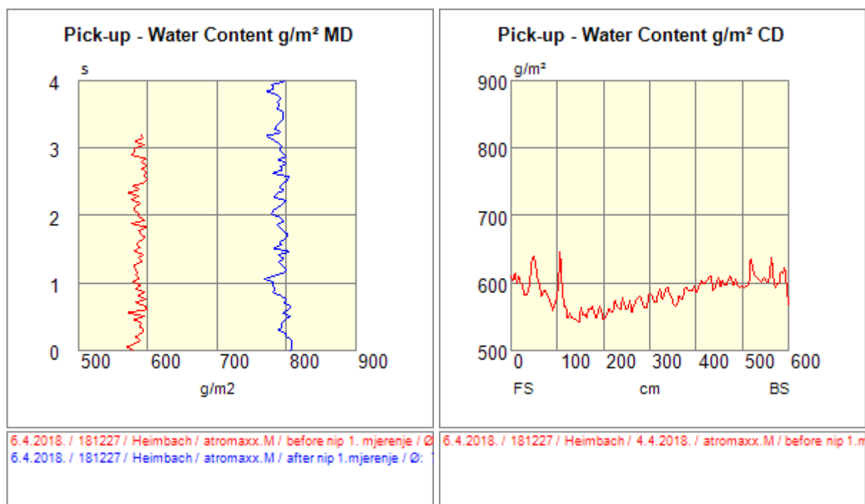
Slika 52. Pick-up filc, prvo mjerenje, MD i CD količine vode
