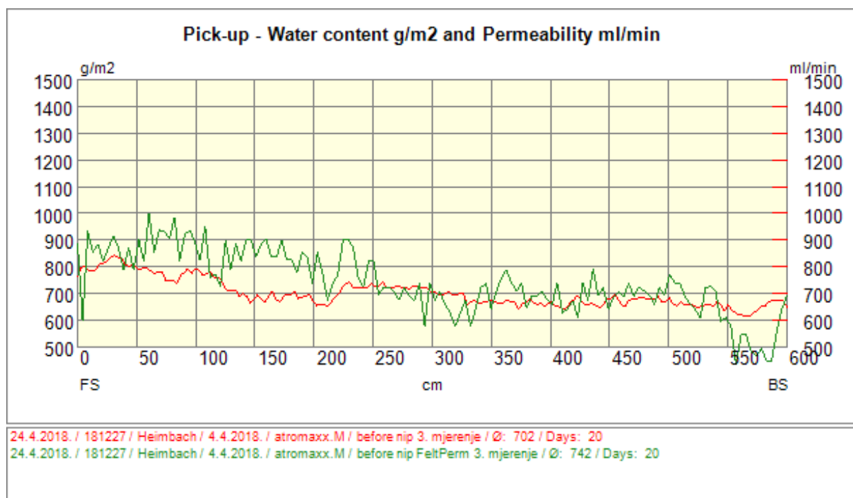
Slika 75. Pick-up ponovljeno, treće mjerenje, CD količina vode i propusnost
