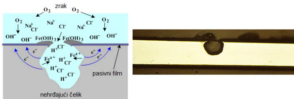
Slika 4. Mehanizam nastanka rupičaste korozije (lijevo); mikrostrukturna snimka u području oštećenja, čelik AISI 304 (EN 1.4301) (desno) [24, 26].
