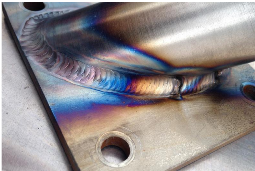
Slika 2. Obojenja površine nastala unosom topline postupkom zavarivanja [16].
