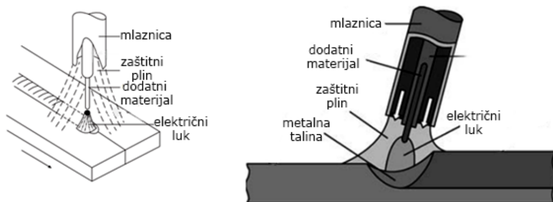
Slika 2.1 MAG zavarivanje
