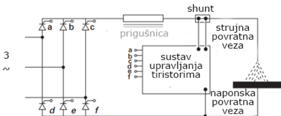
Slika 2.7 Trofazni fazno upravljivi tiristorski ispravljaj u mosnom spoju [6]
