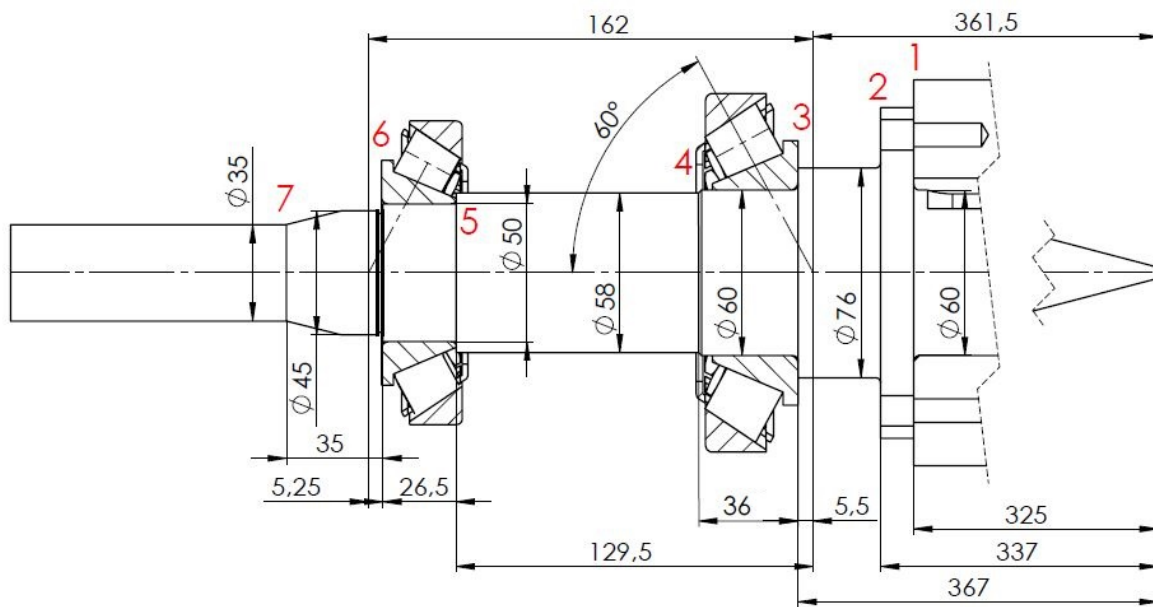
Slika 24. Skica vratila
