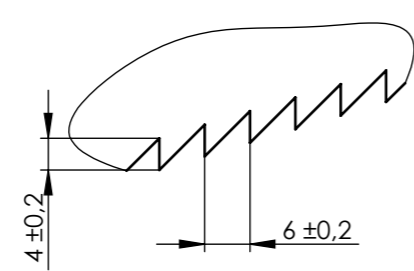
Z (M 5:1)
