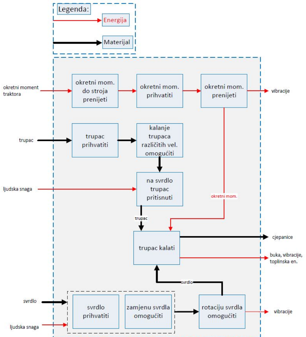
Slika 19. Funkcijska dekompozicija
