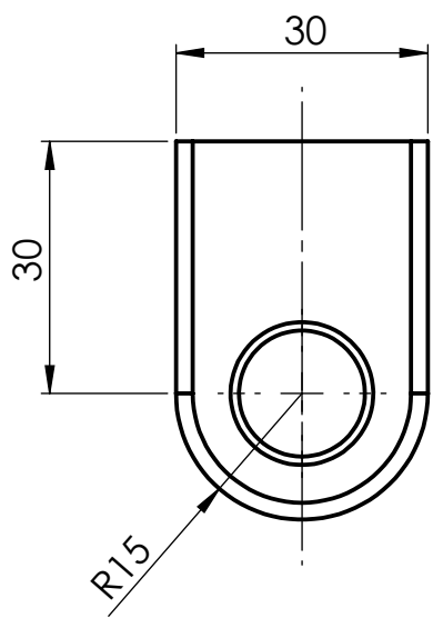
PRESJEK A-A MJERILO 1:1
