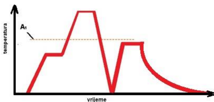
Sl. 26 Dijagram postupka poboljšavanja čelika 100Cr6
