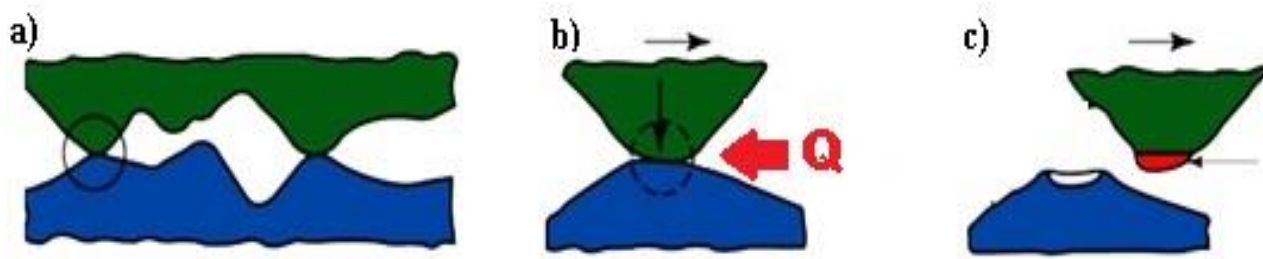
Sl. 8 Shematski prikaz procesa adhezije kroz jedinične događaje [6]
