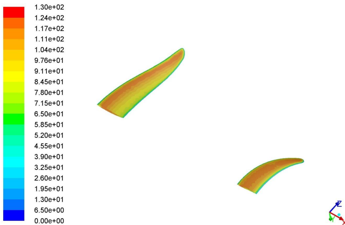
Slika 68. Polje vrijednosti y^+ po površini oba krila, \alpha = 7.5^\circ , v_s = 8 m/s, pogled odozdo
