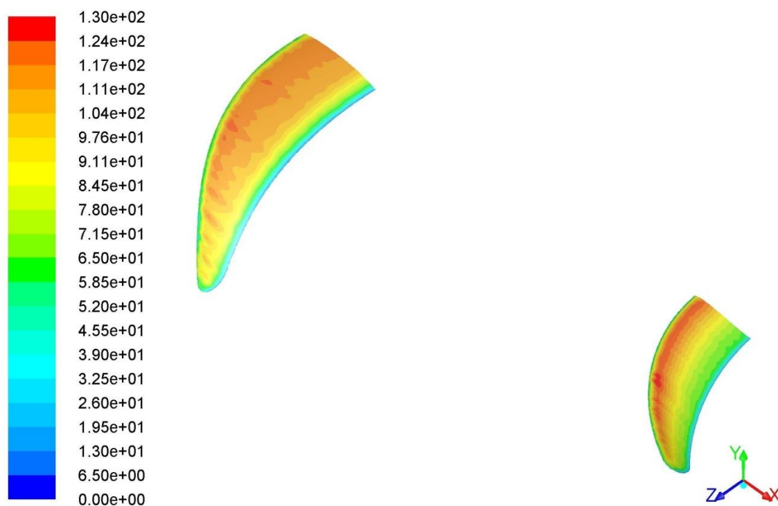
Slika 67. Polje vrijednosti y^+ po površini oba krila, \alpha = 7.5^\circ , v_s = 8 m/s, pogled odozdo
