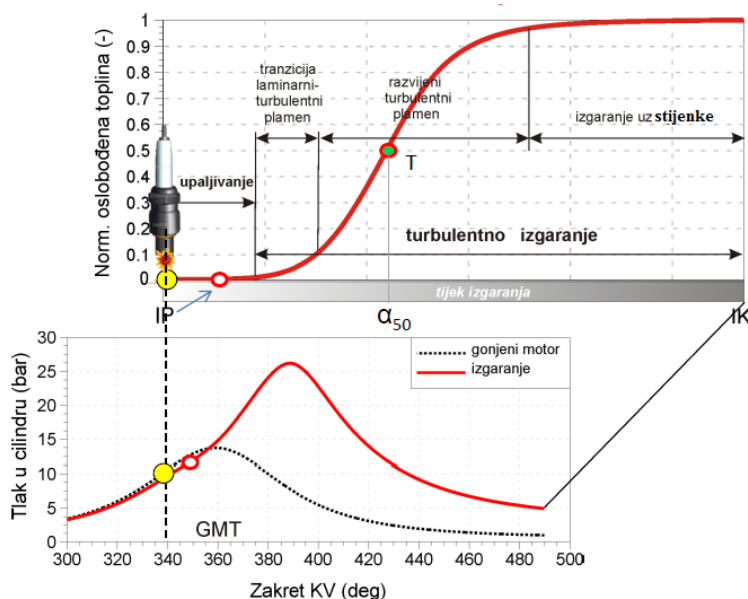
Slika 18. Faze izgaranja u cilindru Ottovog motora [13]
