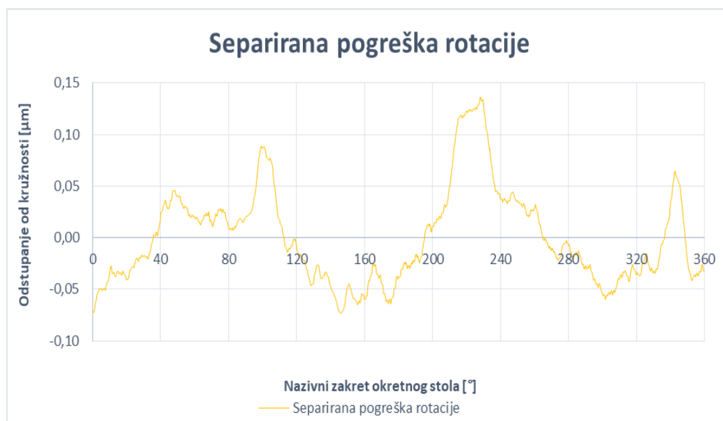
Slika 95. Separirana pogreška rotacije
