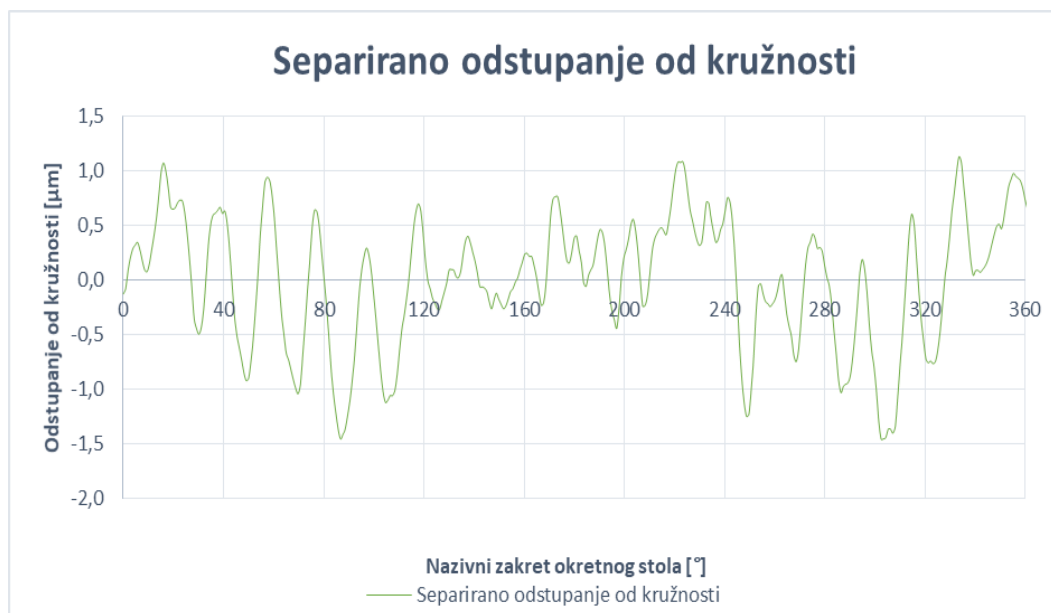
Slika 89. Separirano odstupanje od kružnosti
