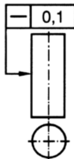
Slika 10. Primjer tolerancije pravocrtnosti [8]
