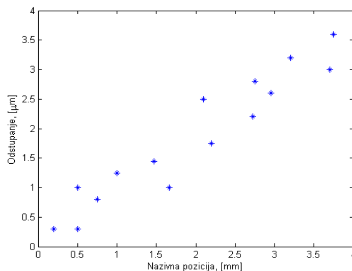
Slika 14. Set podataka mjerenja
