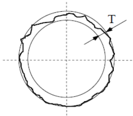
Slika 11. Odstupanje od kružnosti [5]
