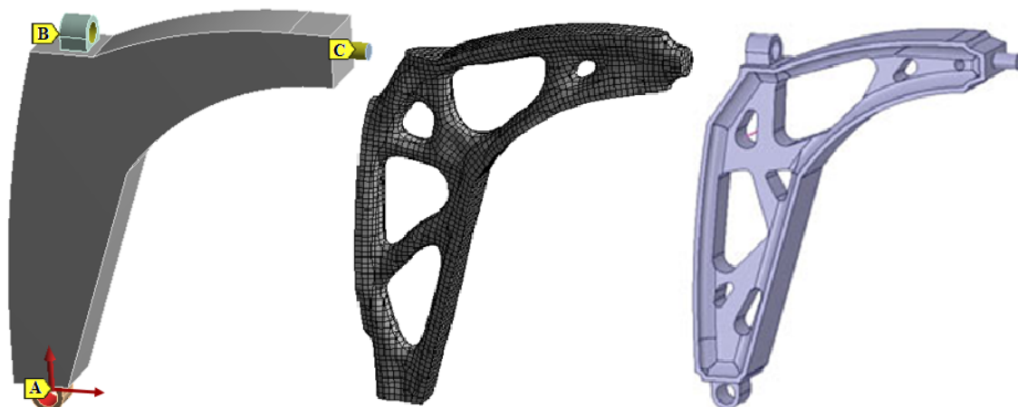
Slika 42. Topološka optimizacija nosača
