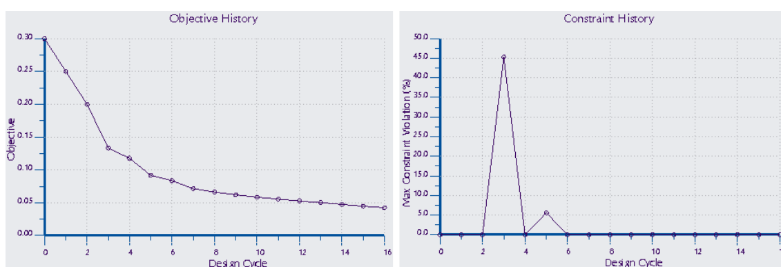
Slika 92. Ovisnost cilja i ograničenja optimizacije topologije o iteraciji (Verzija 5)
