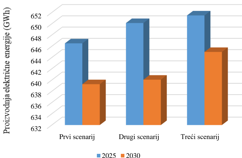
Slika 28. Proizvodnja električne energije po blokovima u 2025. i 2030. godini za sva tri scenarija
