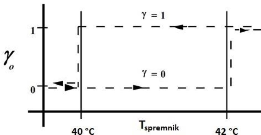
Slika 34. Diferencijalni regulator PTV-a
