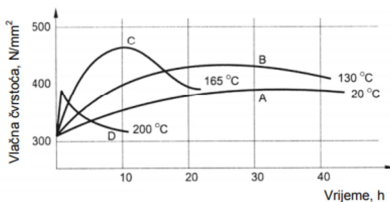
Slika 3. Ovisnost čvrstoće o temperaturi i vremenu dozrijevanja [9]
