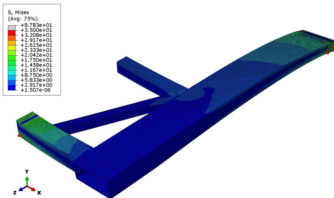
Slika 3.38 – Ekvivalentna von Misesova napreznja [ \text{N/mm}^2 ] 3D modela glavnog nosača za slučaj utovara tereta (kritična mjesta označena su crvenim točkama)
