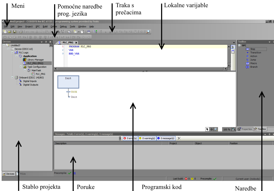
Slika 14. Sučelje Codesys-a
