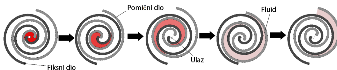
Slika 11. Pužni ekspander [6]
