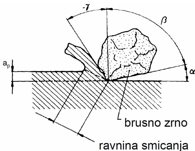
Slika 51 Geometrija rezne oštice brusnog zrna [31]
