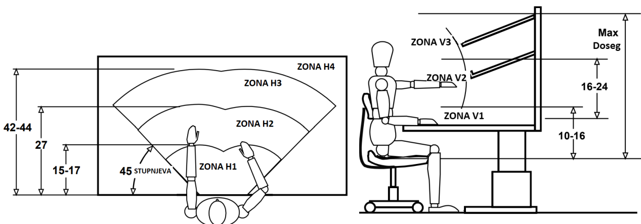
Slika 4.10. Zone doseg [18]
