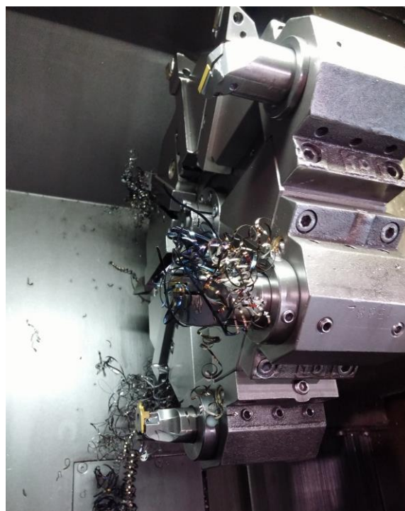
Slika 5.13. Zadržavanje odvojene čestice na reznoj oštreci
