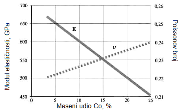
Slika 9. Modul elastičnosti i Poissonov koeficijent kao funkcija udjela Co [5]
