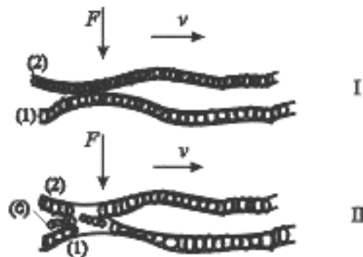
Slika 18. Jedinični događaj oksidacije [7]
